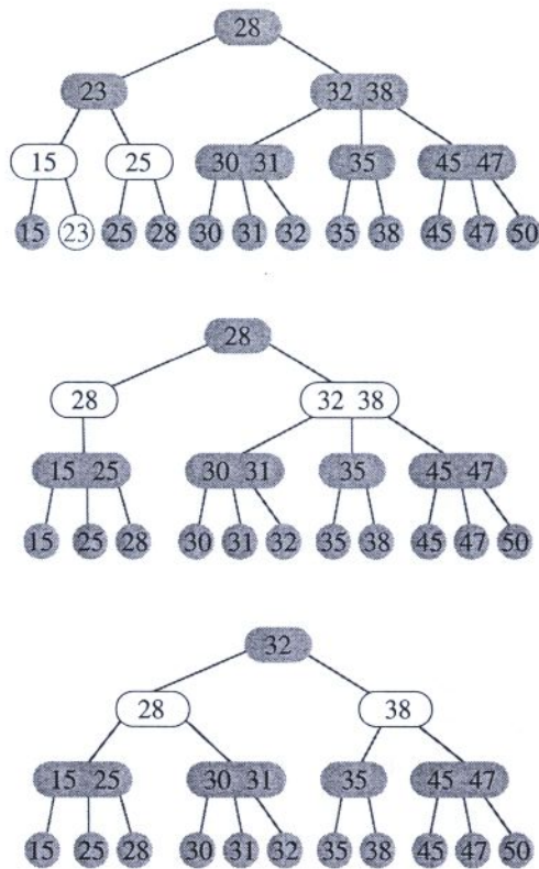
Figura 6.25 Cancellazione del nodo con chiave 23 da un albero 2-3.
