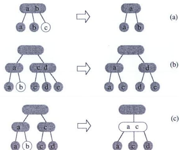
Figura 6.24 Cancellazione da un albero 2-3: vari casi.
