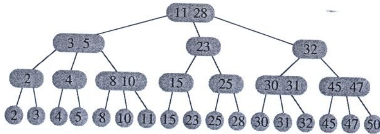
Figura 6.20 Esempio di albero 2-3. I nodi interni con due figli mantengono il massimo del sottoalbero sinistro ( S ); i nodi interni con tre figli mantengono il massimo del sottoalbero sinistro e di quello centrale ( S ed M ).
